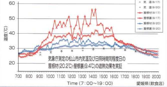
図-1 施工前後の屋根材・屋根裏の温度変化 「ルーフェード」施工前(8/17)赤・施工後(8/20)青の温度変化
