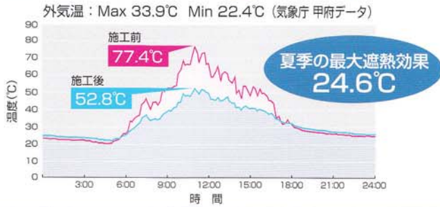
図-2 施工前後の夏季屋根表面温度変化 「ルーフェード」施工前(7/14)赤・施工後(7/14)青の温度変化
