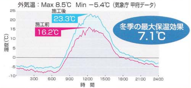
図-3 施工前後の冬季屋根表面温度変化 「ルーフェード」施工前(12/22)赤・施工後(12/22)青の温度変化
